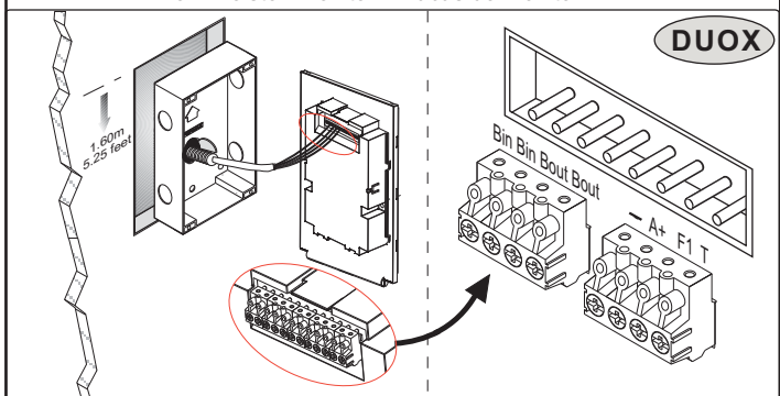
FERMAX iLOFT DUOX 97832 V06_15 Regletas Monitor - Monitor Connectors - Régletes du moniteur Klemmleisten Monitor - Placas do monitor
