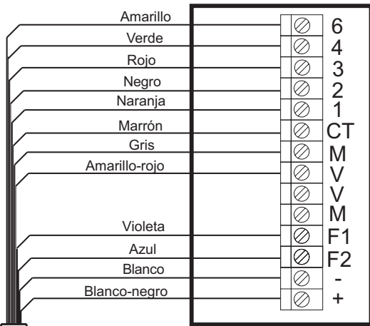
Módulo de conexiones de la peana del monitor Monitor Connection Module Module de Connexions pour le support du moniteur Anschlussmodule für den Monitor
