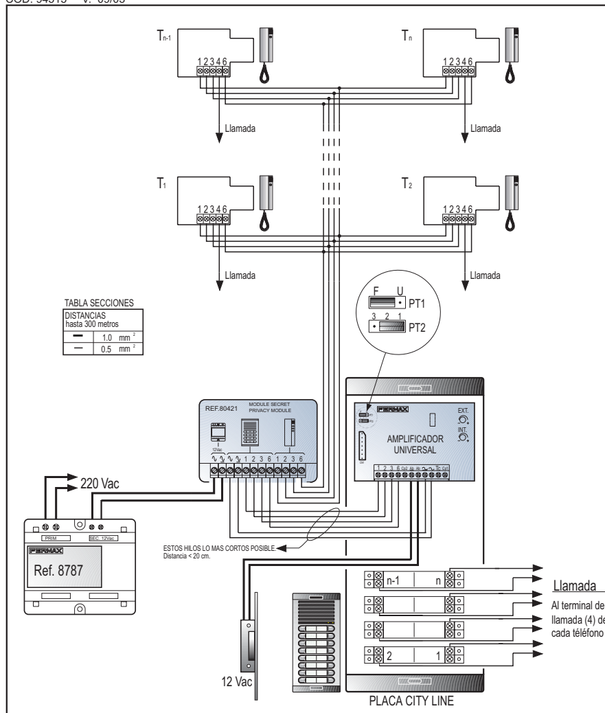
ESQUEMA DE CABLEADO
