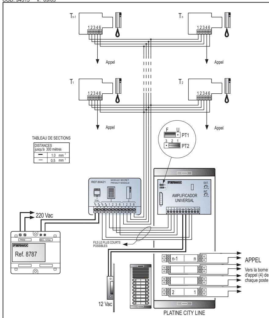
SCHEMA DE CABLAGE
