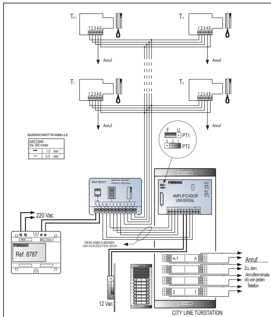
VERKABELUNG DIAGRAM
