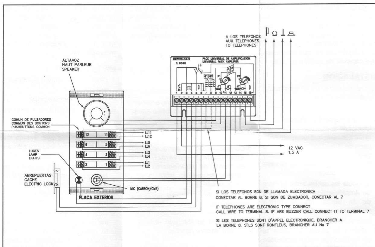
EJEMPLO DE INSTALACION/EXAMPLE DU INSTALLATION/EXAMPLE OF INSTALLATION
